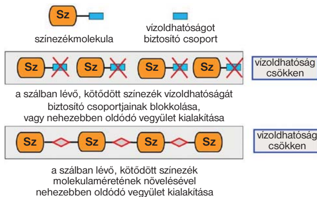
4. ábra. A nedves szintartótságot növelő utánkezelések, vázlatosan
