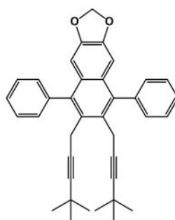
17. ábra. Egy naftálember és Spartan programmal meghatározott szerkezete
